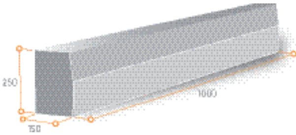
CESTOVNI RUBNICI . road curbs
